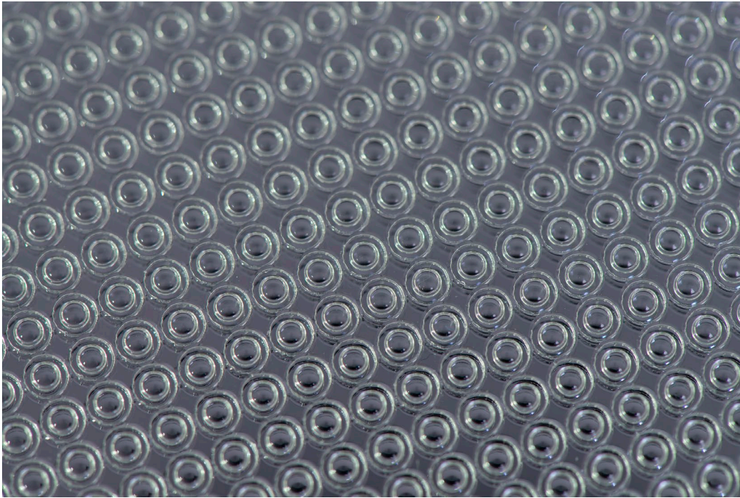
圖二_針對晶圓級光學技術 300mm 步進重複母模特寫
